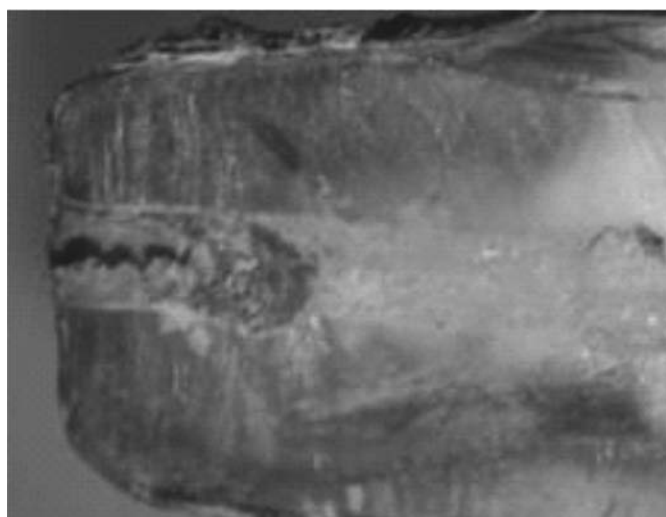
Figura 5. Espécime do grupo Histoacryl® (Laboratório B. Braun do Brasil, São Gonçalo, Brasil), não apresentando penetração linear de Rodamina B (0.000 mm).
